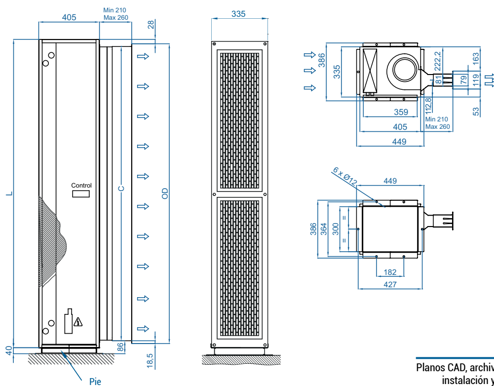
Instalación vertical
