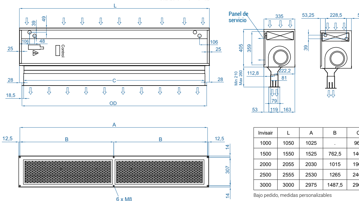
Instalación horizontal
