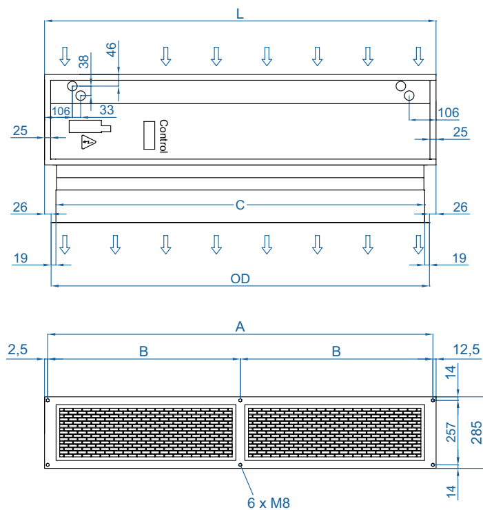
Instalación horizontal
